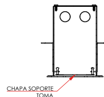
CORTE MODELO SALIENTE EDIFICIO E PARED 120mm / ARTEFACTO 170mm ESC. 1:8
