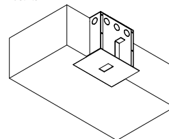
CORTE MODELO EMPOTRADO EDIFICIO F PARED 160mm / ARTEFACTO 160mm ESC. 1:8
