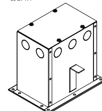
AXONOMETRIA TRASERA ESC. 1:4
