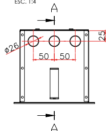
VISTA TRASERA ESC. 1:4
