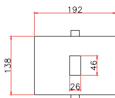
VISTA LATERAL ESC. 1:4
