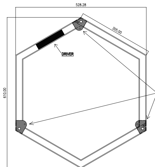
SOPORTE PARA PLAFON
